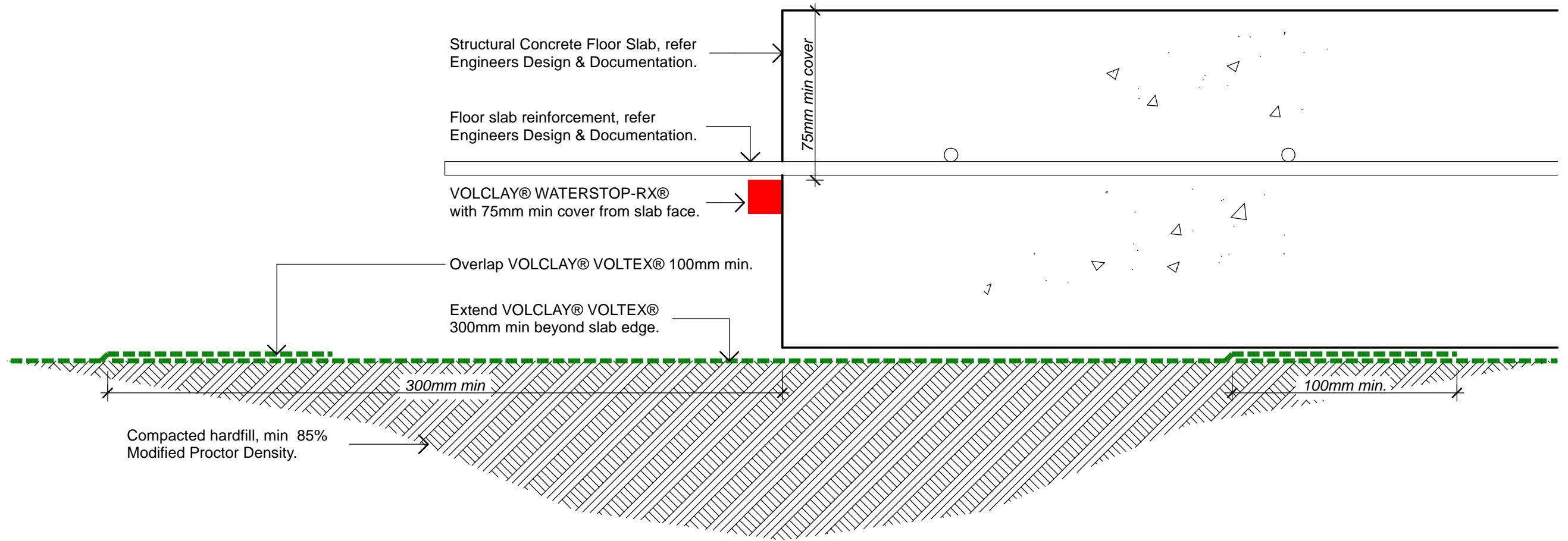
Cold Pour Construction Joint Scale 1:2 (A3)
